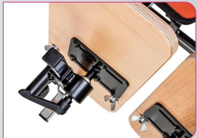
Fußplatten mit Kugelgelenk für SpitzfußEinstellung footplate with ball joint for angle adjustable
