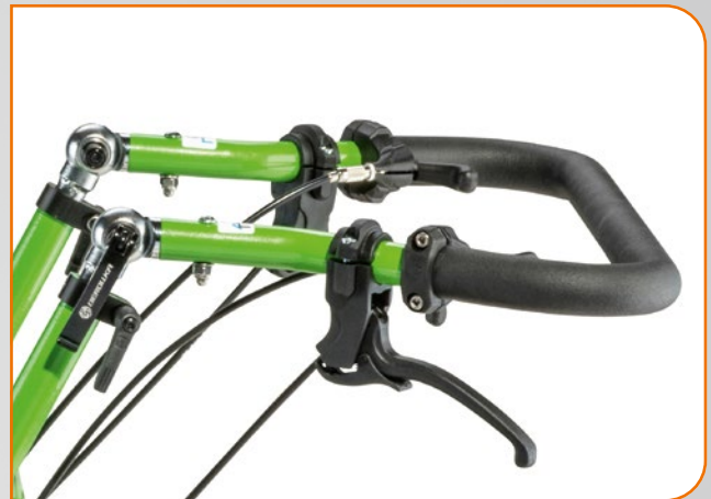
Handbogen, höhen- und winkelverstellbar und abklappbar handbow, height and angle adjustable and foldable
