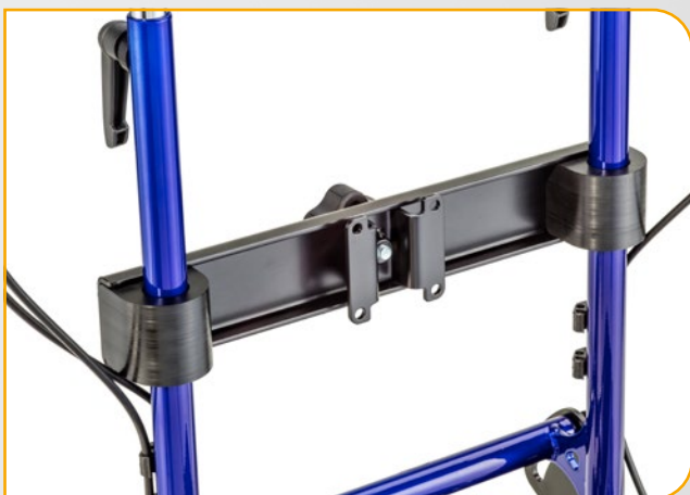
Rückenführung mittig mit Gleitbuchse am Rückenrohr central back shell adaption with slide bushing on back frame
