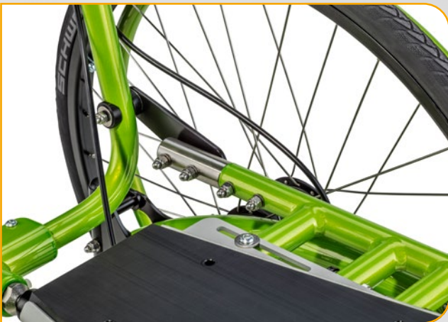
Sitzverlängerung (+7 cm nach hinten) seat extension (+7cm backwards)
